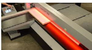
Statusanzeige rot: Achtung, Druckbalken senkt sich
