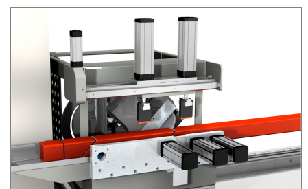
Horizontale und vertikale Spanneinrichtungen 04
